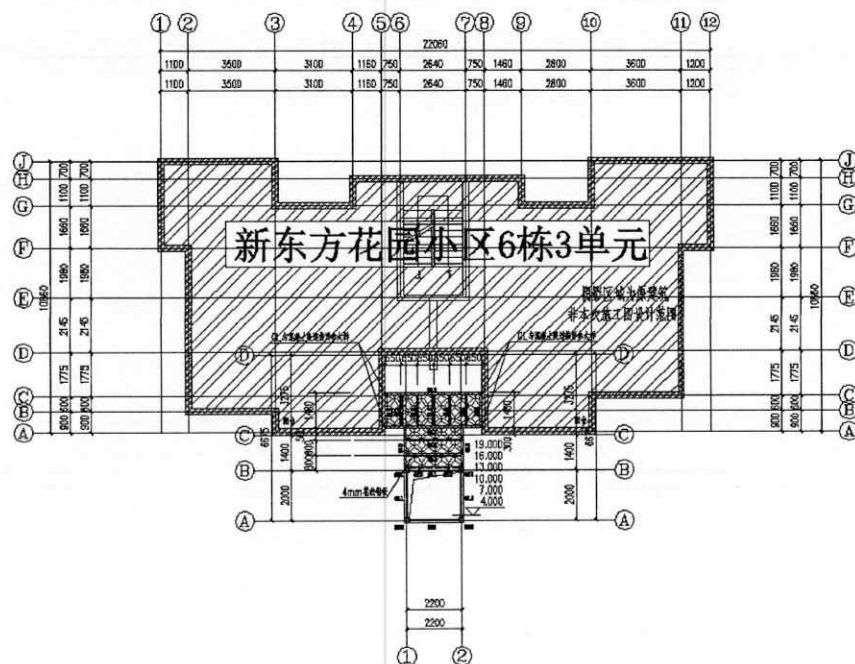
图 2-1 新增电梯标准层结构平面布置
