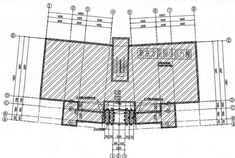
图 2-1 新增电梯标准层结构平面布置
