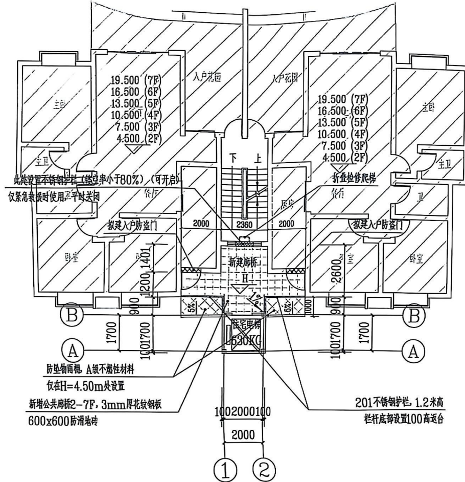
新增电梯标准层 (2-7层) 平面布置图 1:150
