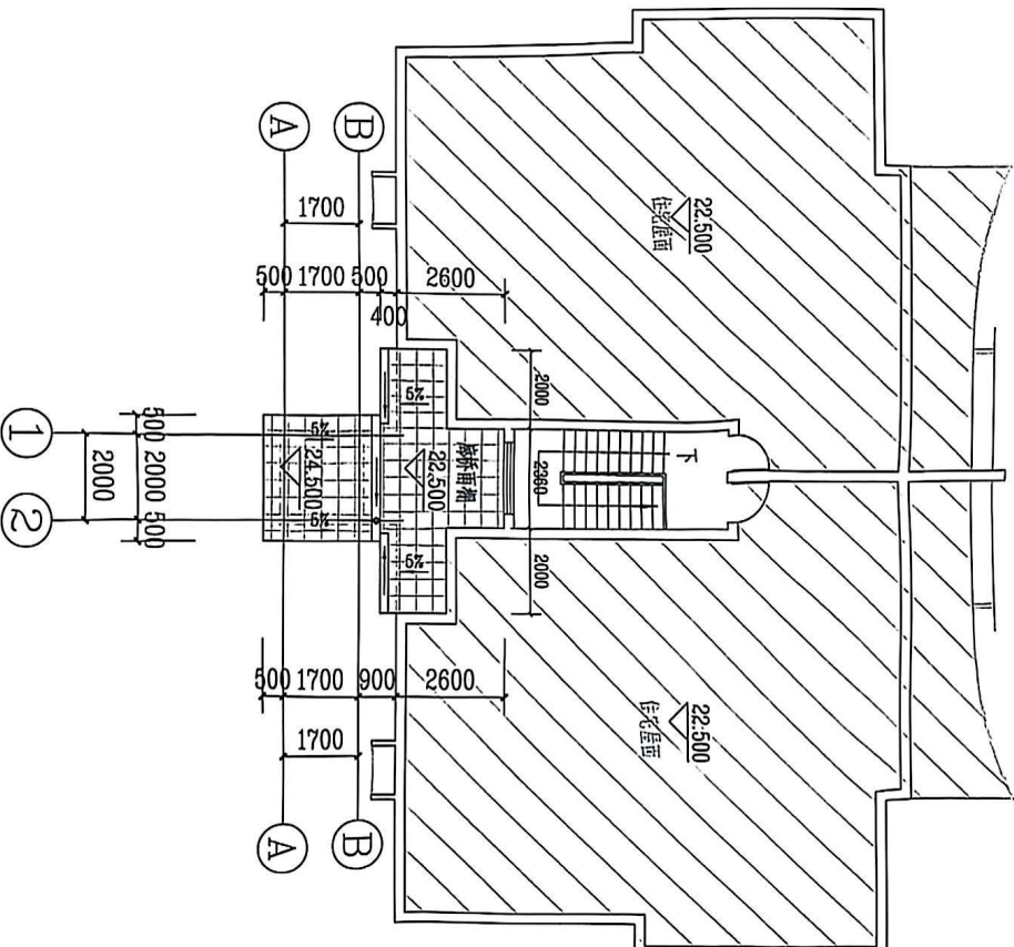
新增电梯屋顶层平面布置图 1:150
