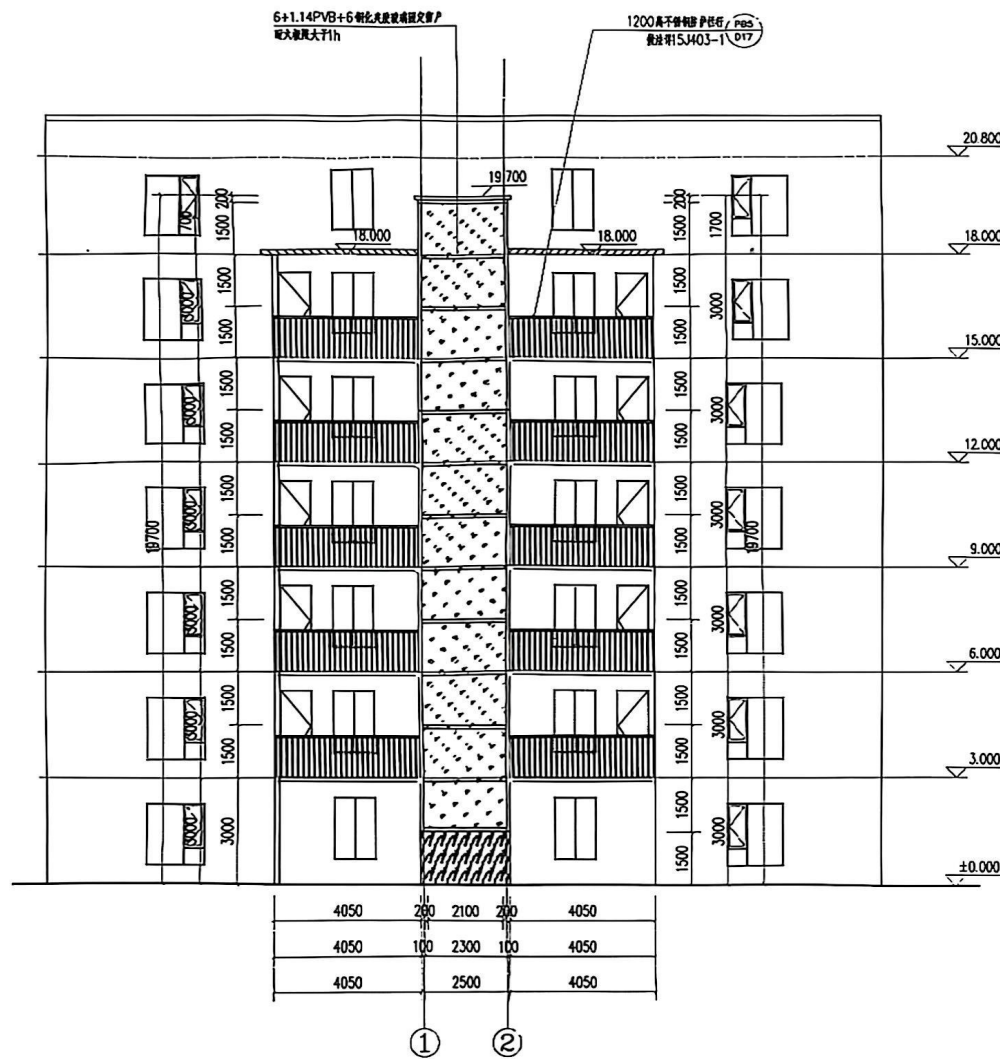
立面图一
