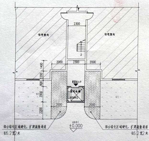
新增电梯首层平面图
