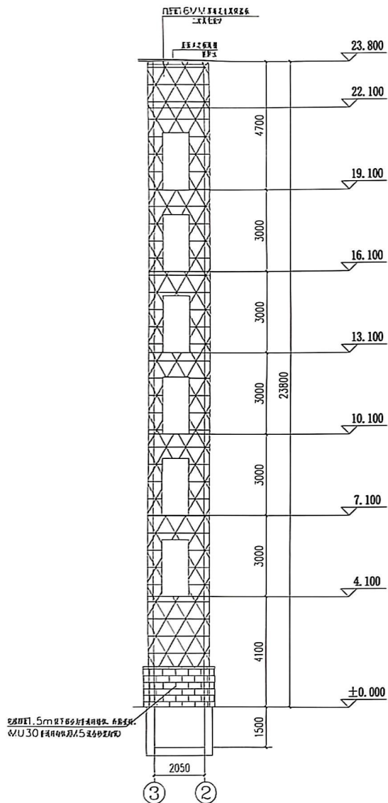
电梯3-2轴立面图 1:100
