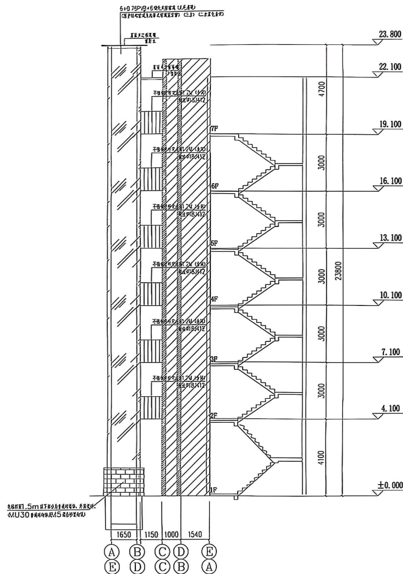
电梯A-E/E-A轴立面图 1:100
