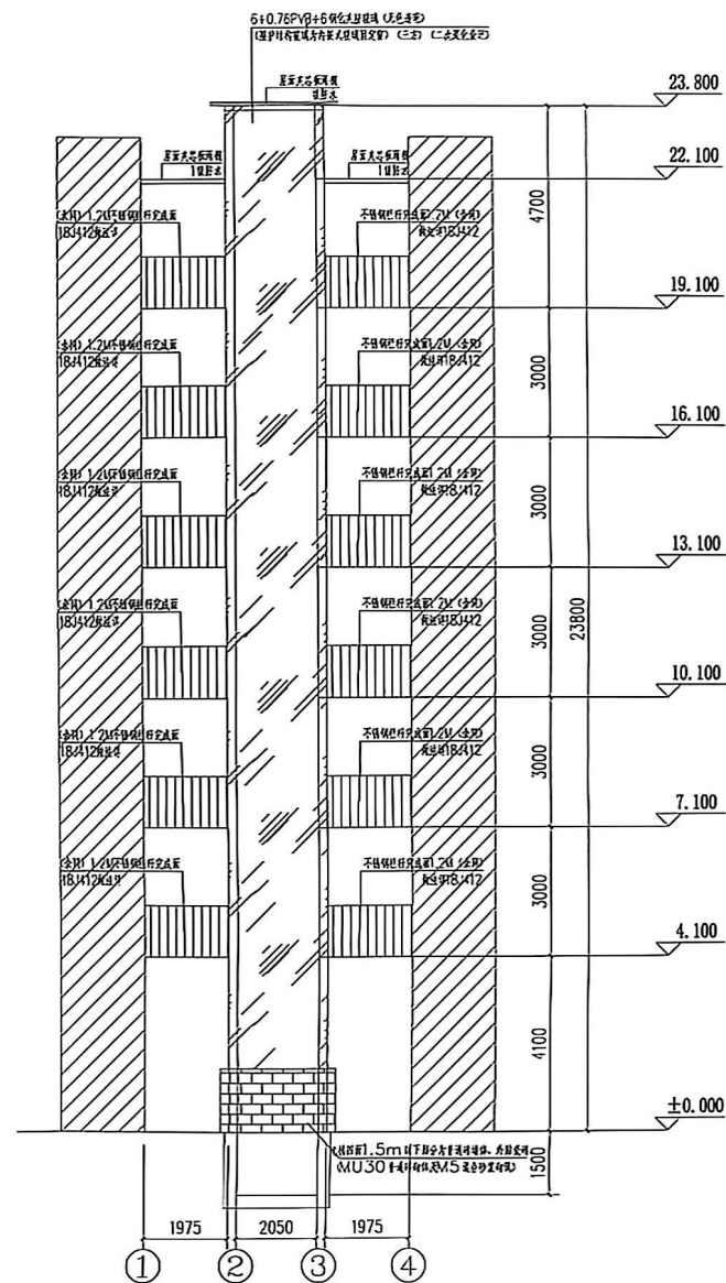
电梯3-2轴立面图 1:100
