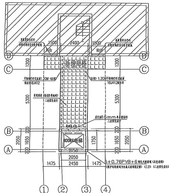
三至七层平面图 1:100
