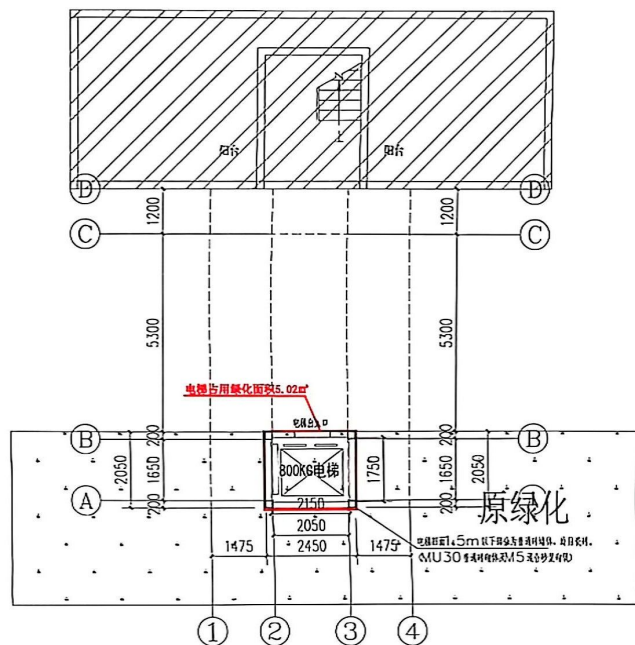
一层平面图 1:100
