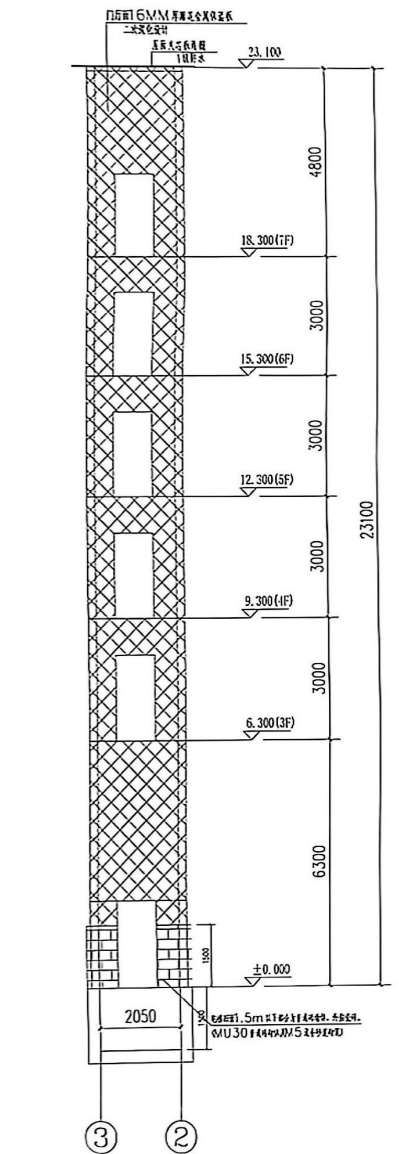
3-2轴立面图 1:100
