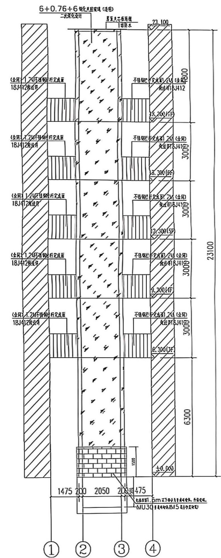
1-4轴立面图 1:100
