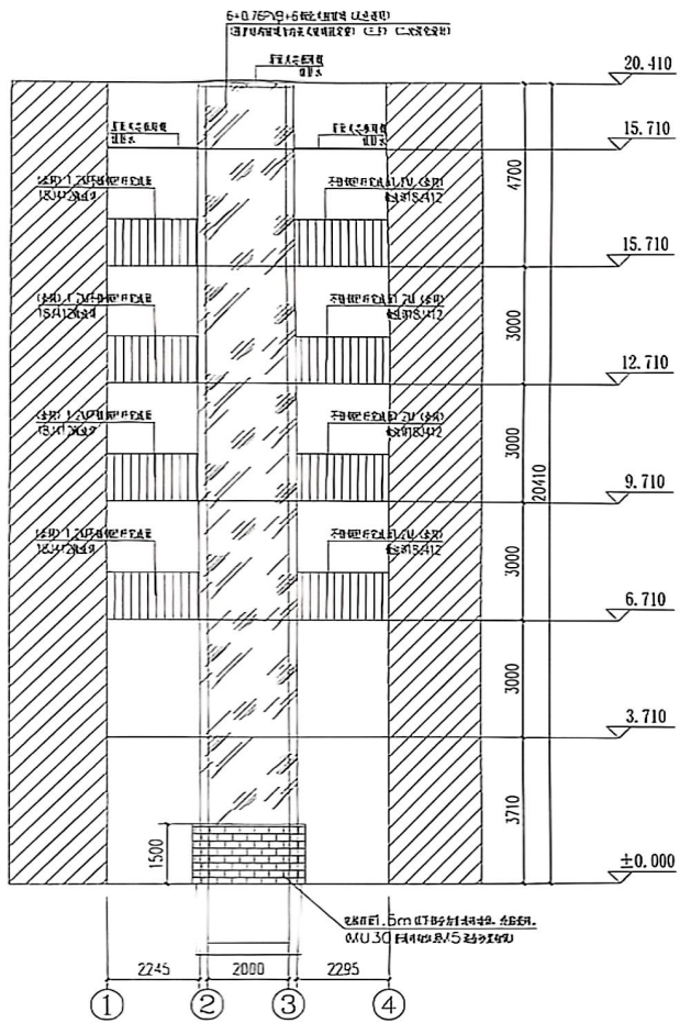
电梯1-4轴立面图 1:100
