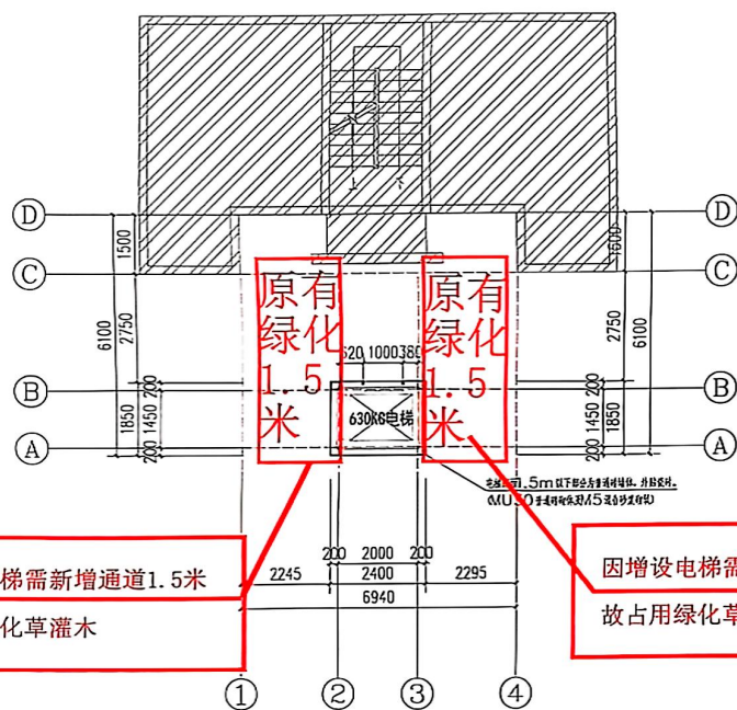
一层平面图 1:100
