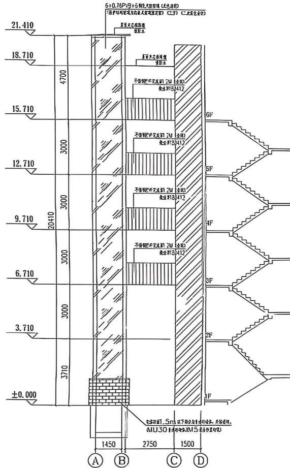
电梯A-D/D-A轴立面图 1:100
