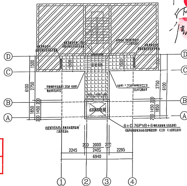
三-六层平面图 1:100
