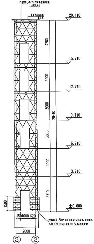
电梯3-2轴立面图 1:100
