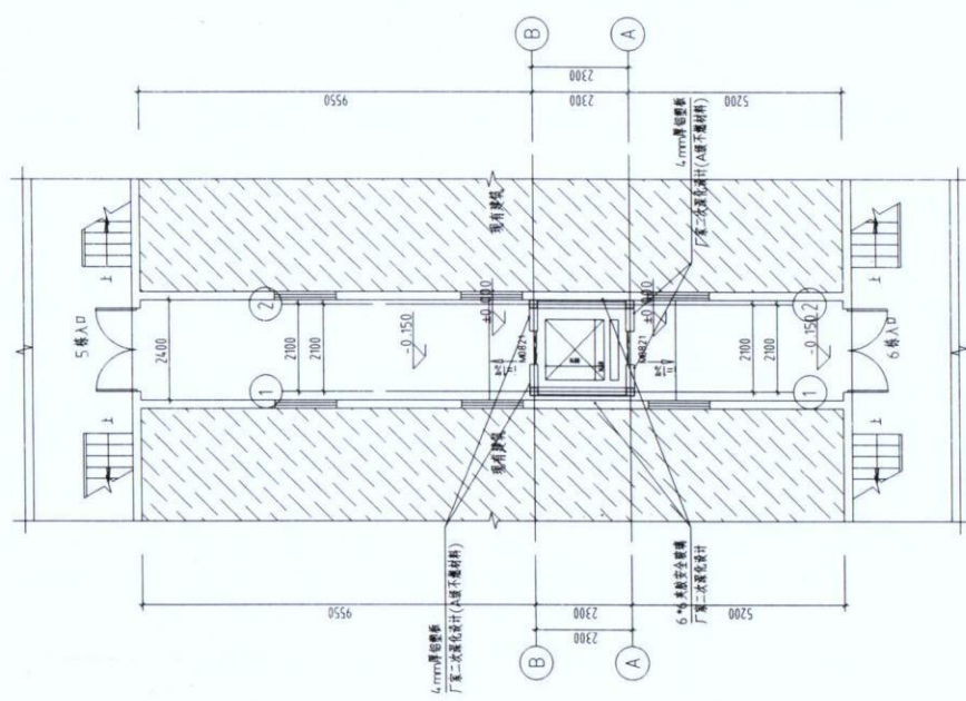
6樓二八層平面圖 比例尺: 1:100
