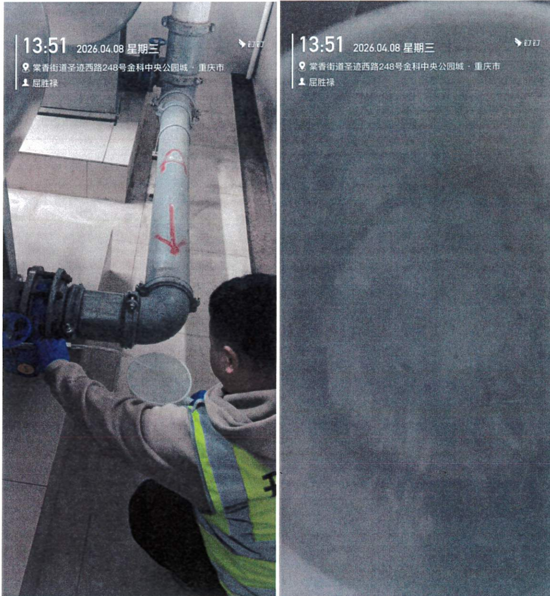
F1:金科中央公园城三期负一楼水泵房 (西门水厂二次供水)
